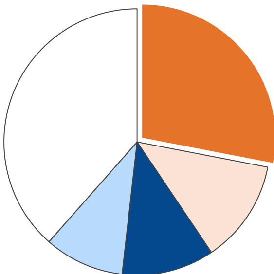
業務部門・エネルギー消費量合計 77 TJ
