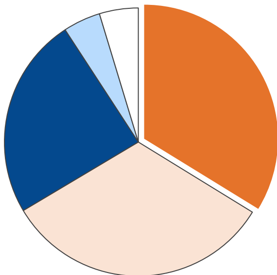
産業部門・エネルギー消費量合計 263 TJ
