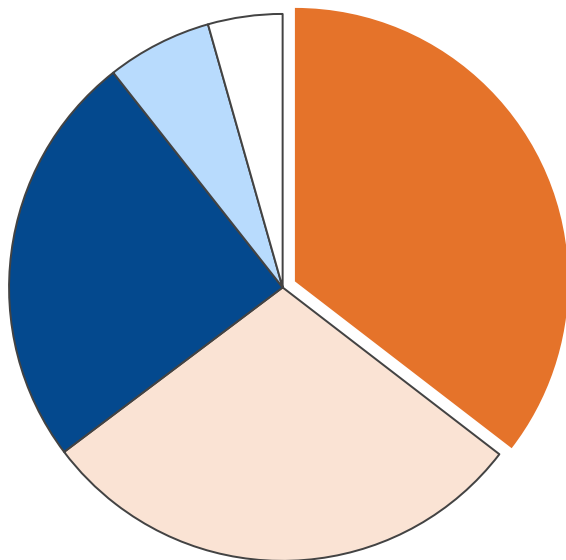
産業部門・二酸化炭素排出量合計 18,239 t-CO 2
