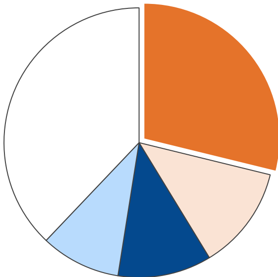
業務部門・二酸化炭素排出量合計 4,902 t-CO 2
