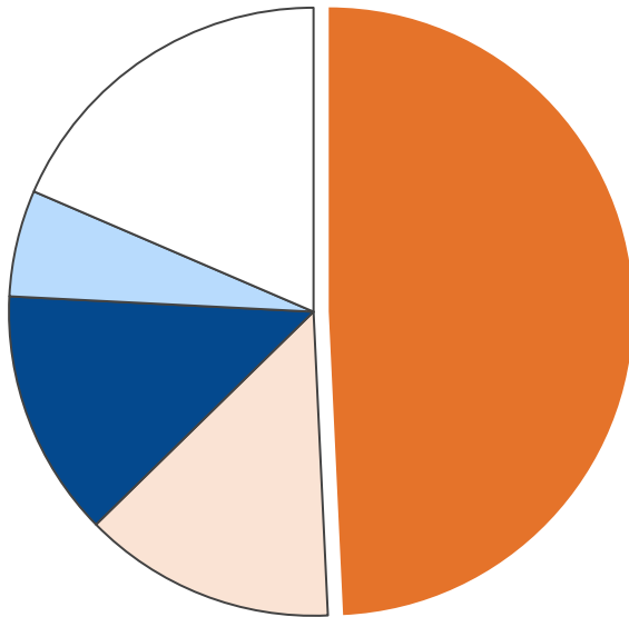
業務部門・二酸化炭素排出量合計 3,333 t-CO 2
