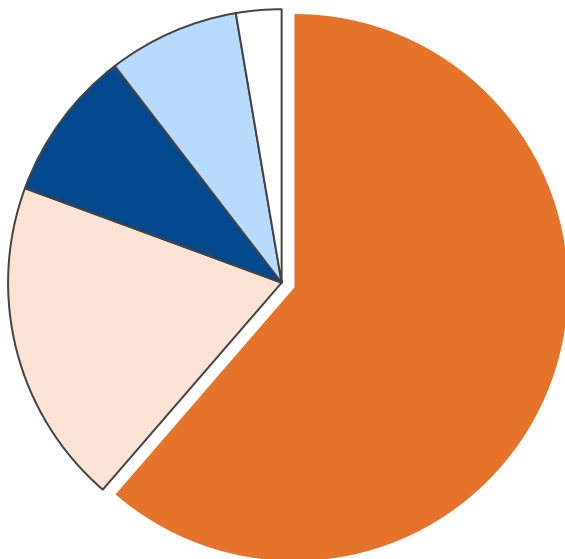
産業部門・エネルギー消費量合計 50 TJ
