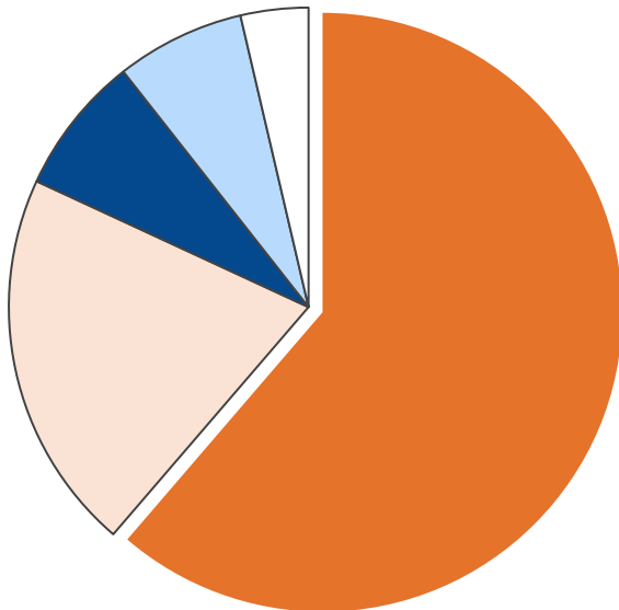
産業部門・二酸化炭素排出量合計 3,485 t-CO 2
