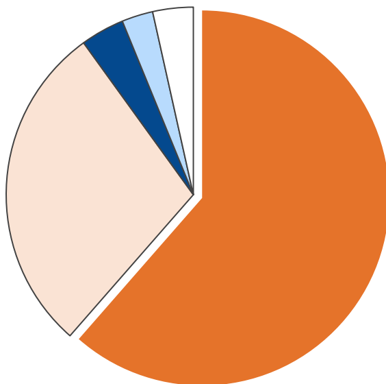
産業部門・エネルギー消費量合計 310 TJ
