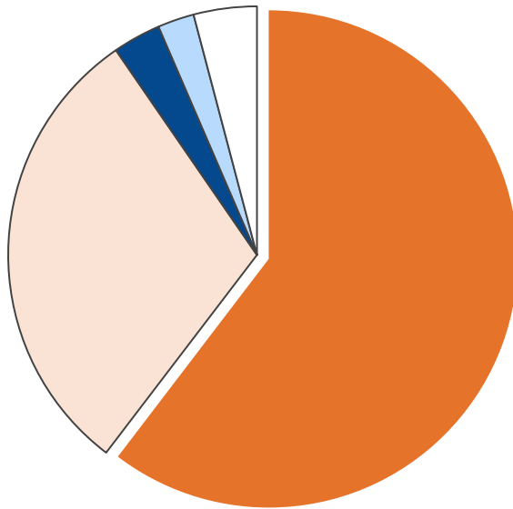
産業部門・二酸化炭素排出量合計 22,117 t-CO 2
