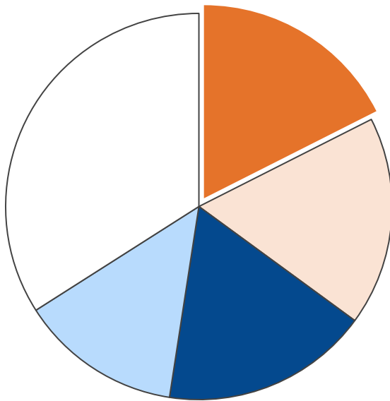
業務部門・二酸化炭素排出量合計 3,131 t-CO 2
