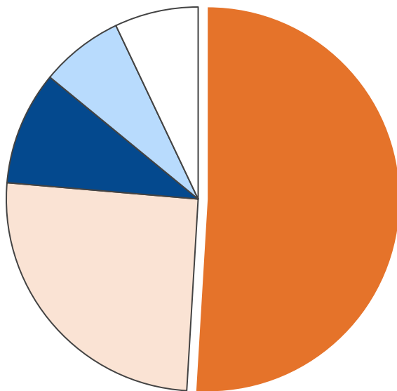
産業部門・二酸化炭素排出量合計 30,749 t-CO 2
