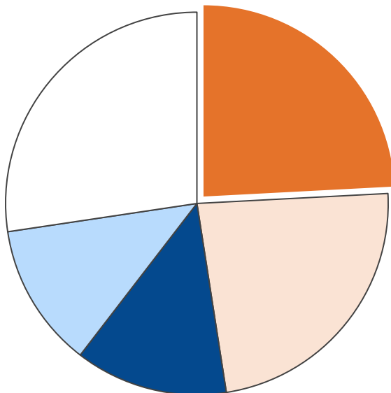
業務部門・エネルギー消費量合計 231 TJ
