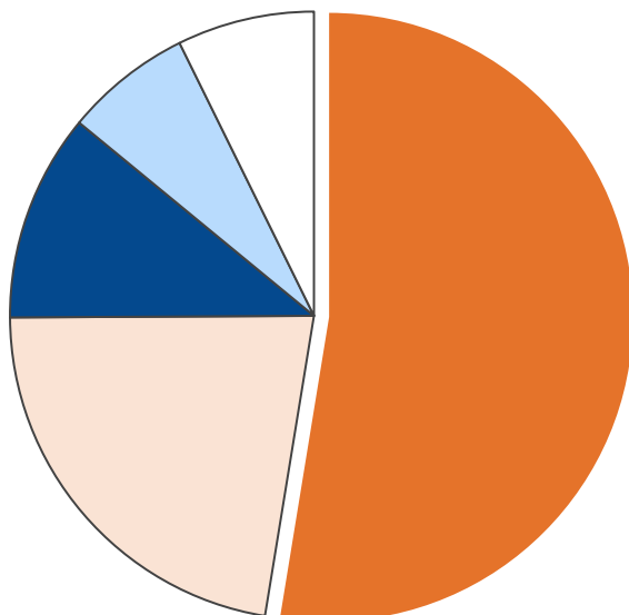
産業部門・エネルギー消費量合計 425 TJ
