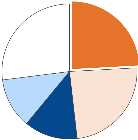
業務部門・二酸化炭素排出量合計 14,719 t-CO 2
