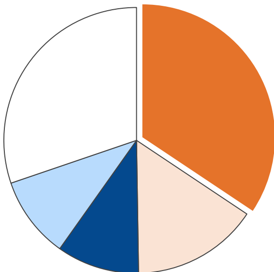
業務部門・エネルギー消費量合計 45 TJ
