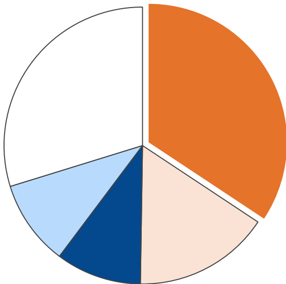
業務部門・二酸化炭素排出量合計 2,867 t-CO 2
