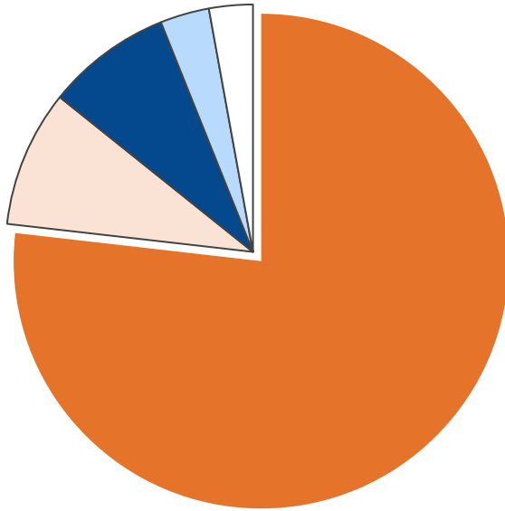
産業部門・二酸化炭素排出量合計 3,071 t-CO 2
