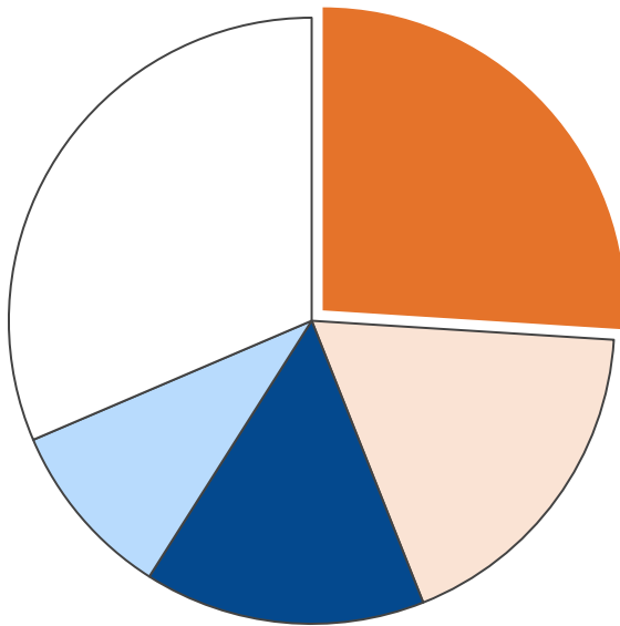
業務部門・二酸化炭素排出量合計 69,893 t-CO 2
