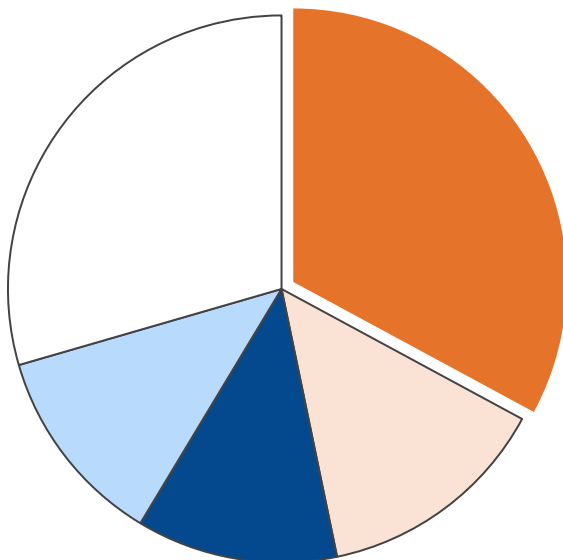
産業部門・エネルギー消費量合計 1,510 TJ
