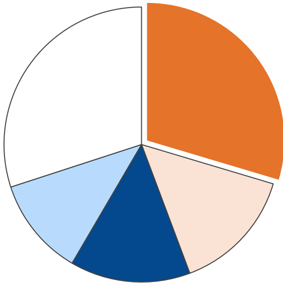
産業部門・二酸化炭素排出量合計 98,867 t-CO 2
