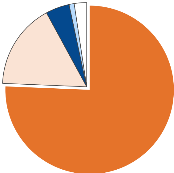
産業部門・エネルギー消費量合計 2,722 TJ
