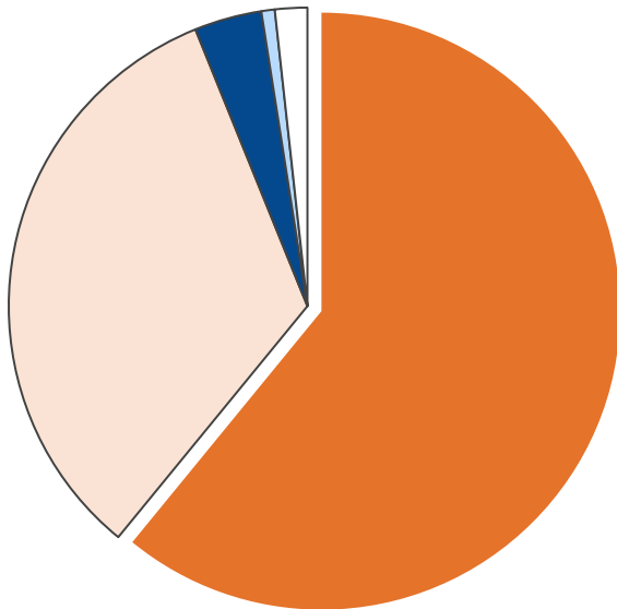
産業部門・二酸化炭素排出量合計 202,152 t-CO 2
