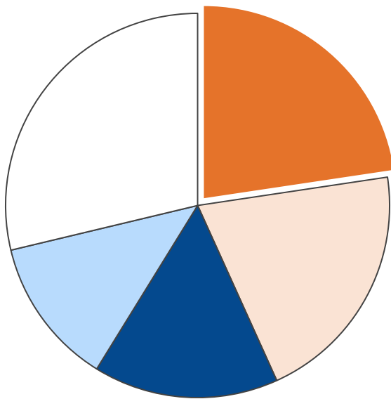
業務部門・二酸化炭素排出量合計 9,751 t-CO 2
