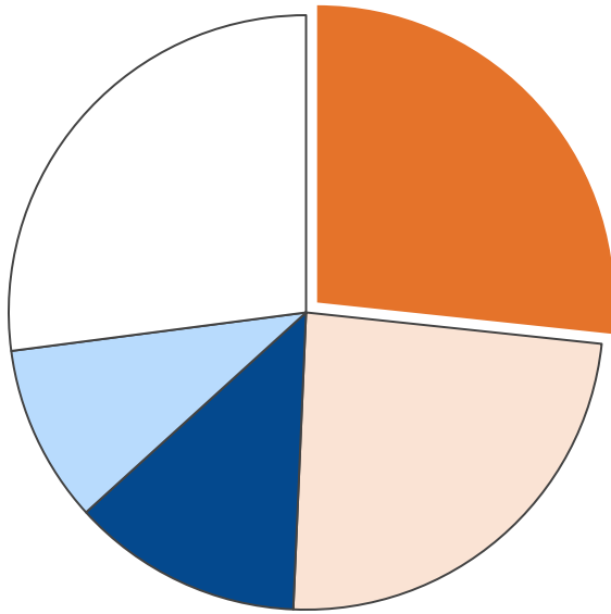
業務部門・二酸化炭素排出量合計 36,975 t-CO2
