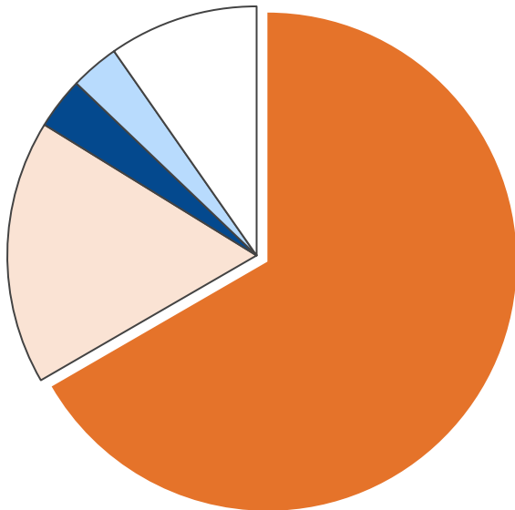
産業部門・二酸化炭素排出量合計 127,464 t-CO 2
