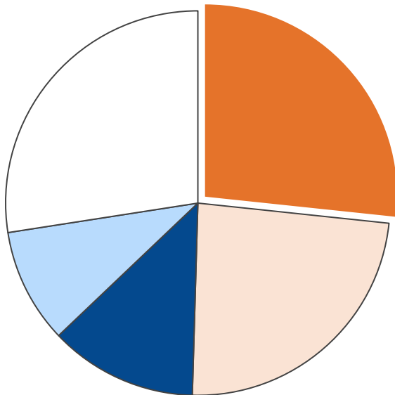
業務部門・エネルギー消費量合計 624 TJ
