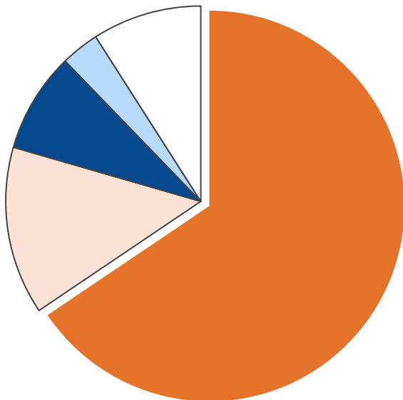
産業部門・エネルギー消費量合計 2,285 TJ
