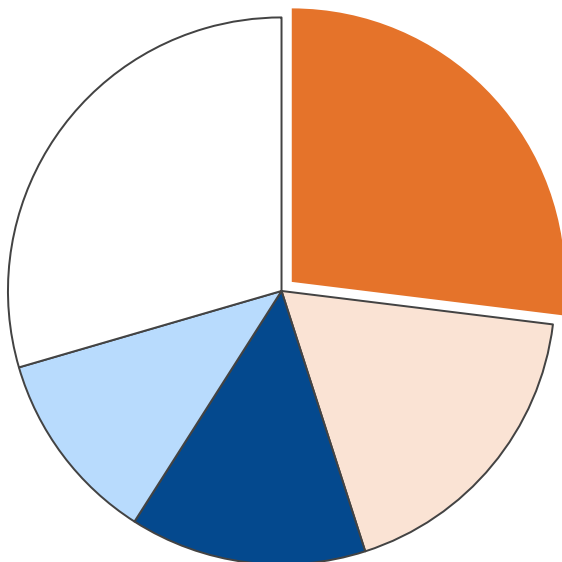
業務部門・エネルギー消費量合計 865 TJ
