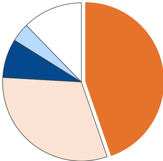
産業部門・二酸化炭素排出量合計 171,927 t-CO 2
