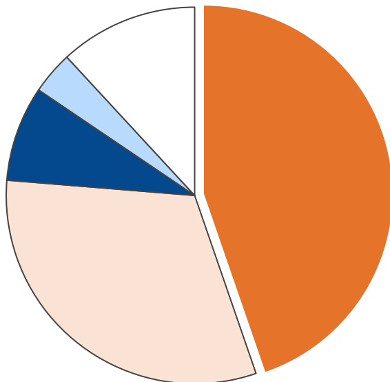
産業部門・エネルギー消費量合計 2,824 TJ
