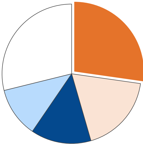
業務部門・二酸化炭素排出量合計 51,196 t-CO 2
