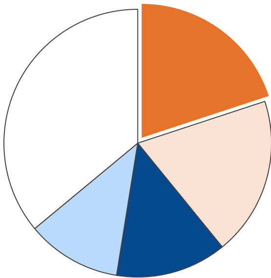
産業部門・二酸化炭素排出量合計 23,498 t-CO 2
