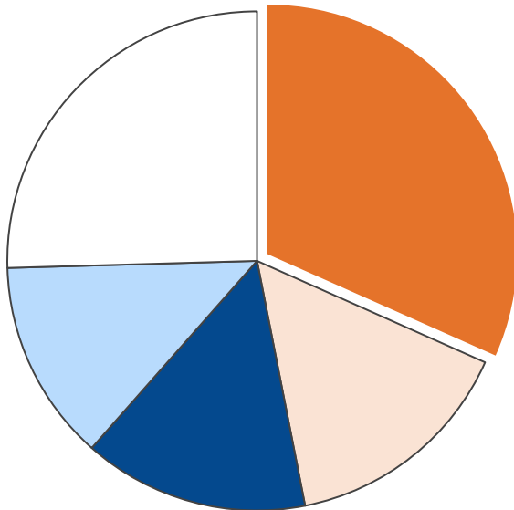
業務部門・エネルギー消費量合計 272 TJ
