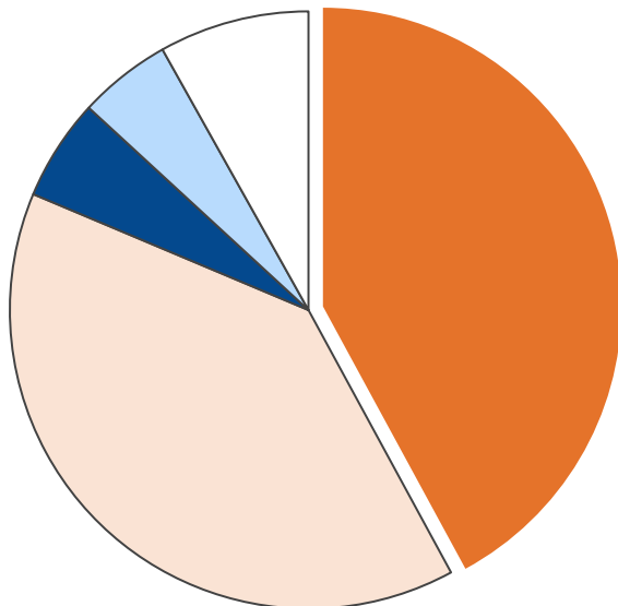
産業部門・エネルギー消費量合計 365 TJ
