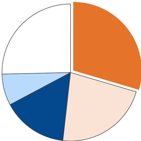
業務部門・二酸化炭素排出量合計 12,543 t-CO 2
