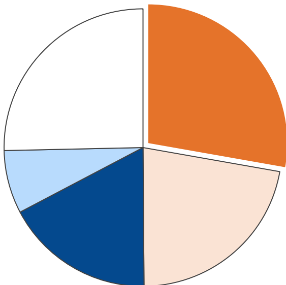
業務部門・エネルギー消費量合計 211 TJ
