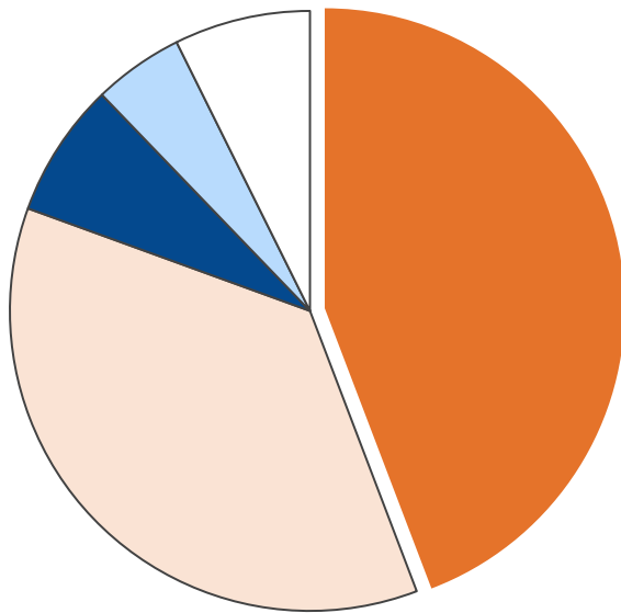
産業部門・二酸化炭素排出量合計 23,869 t-CO 2
