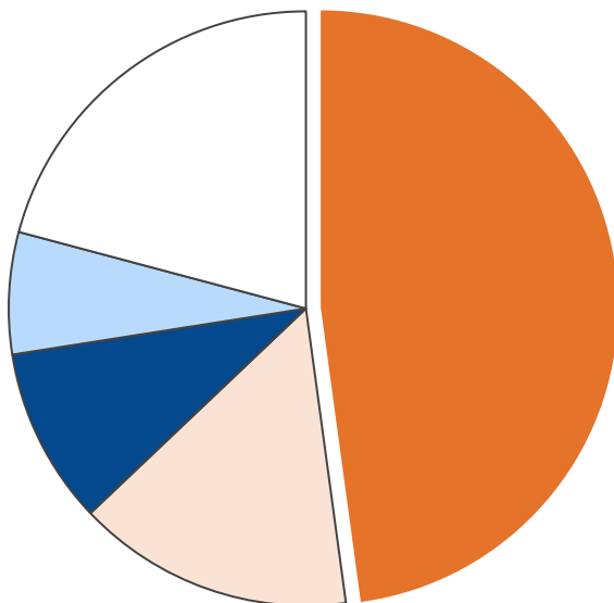
産業部門・エネルギー消費量合計 8,477 TJ
