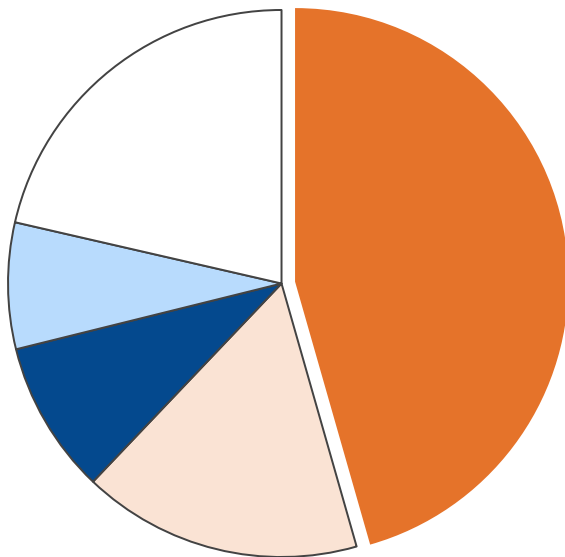
産業部門・二酸化炭素排出量合計 516,998 t-CO 2
