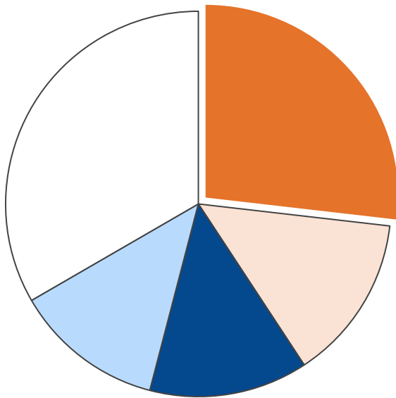
業務部門・二酸化炭素排出量合計 101,288 t-CO 2
