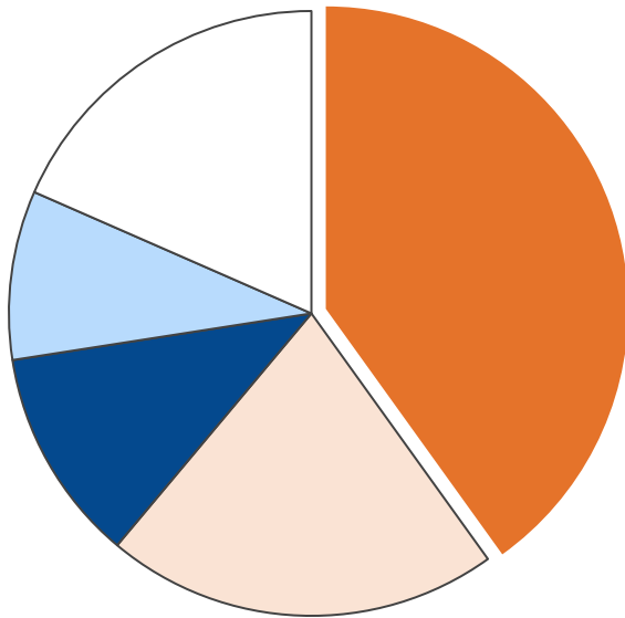
産業部門・二酸化炭素排出量合計 19,677 t-CO 2
