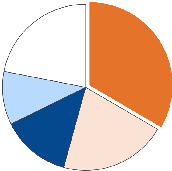
業務部門・二酸化炭素排出量合計 8,225 t-CO 2
