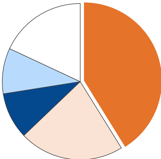
産業部門・エネルギー消費量合計 351 TJ
