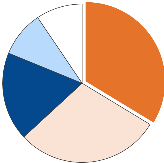
産業部門・二酸化炭素排出量合計 361,670 t-CO 2
