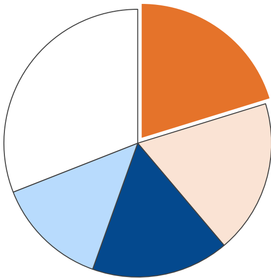
業務部門・二酸化炭素排出量合計 123,534 t-CO 2
