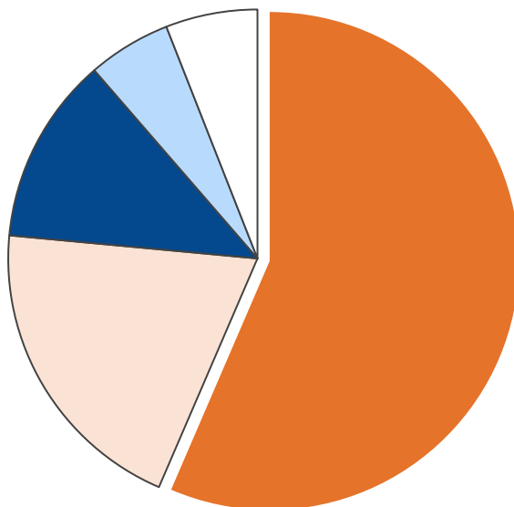
産業部門・エネルギー消費量合計 9,742 TJ
