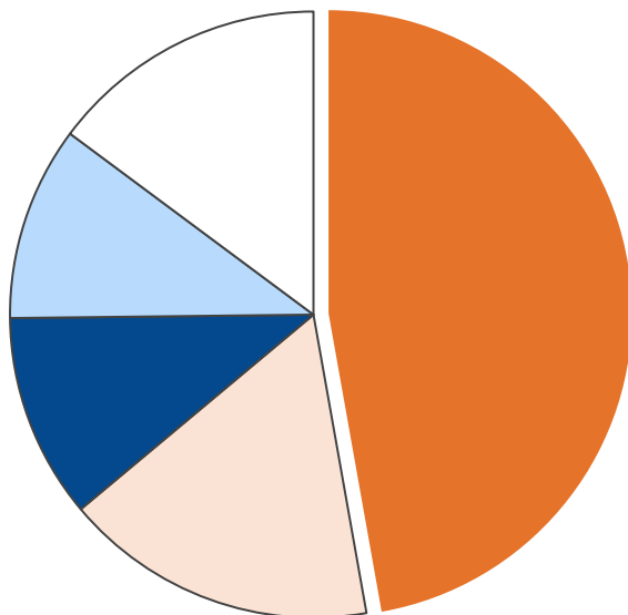
産業部門・エネルギー消費量合計 10,502 TJ
