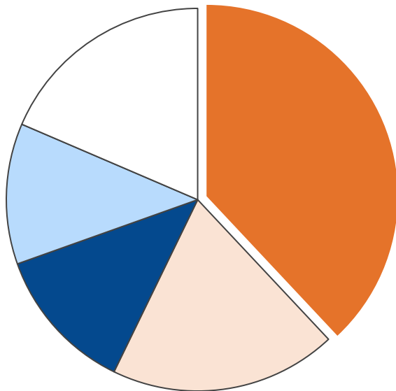
産業部門・二酸化炭素排出量合計 505,750 t-CO 2
