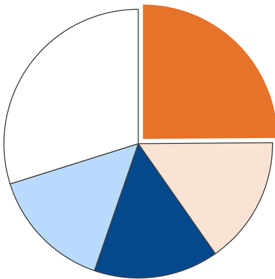
業務部門・二酸化炭素排出量合計 112,429 t-CO 2
