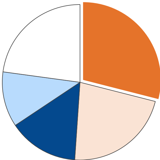
産業部門・二酸化炭素排出量合計 236,075 t-CO 2
