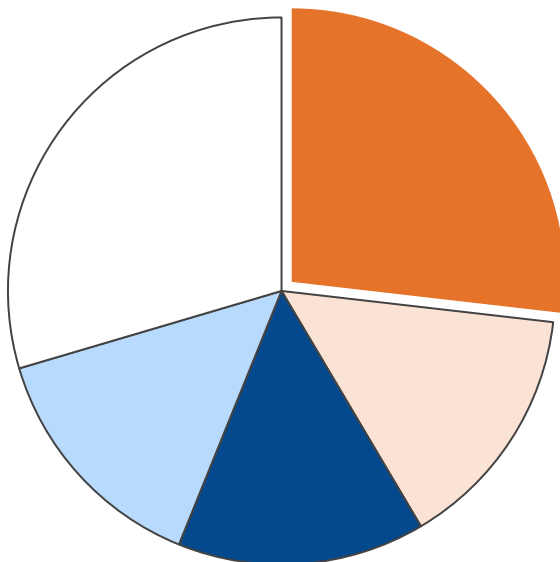
業務部門・エネルギー消費量合計 2,766 TJ
