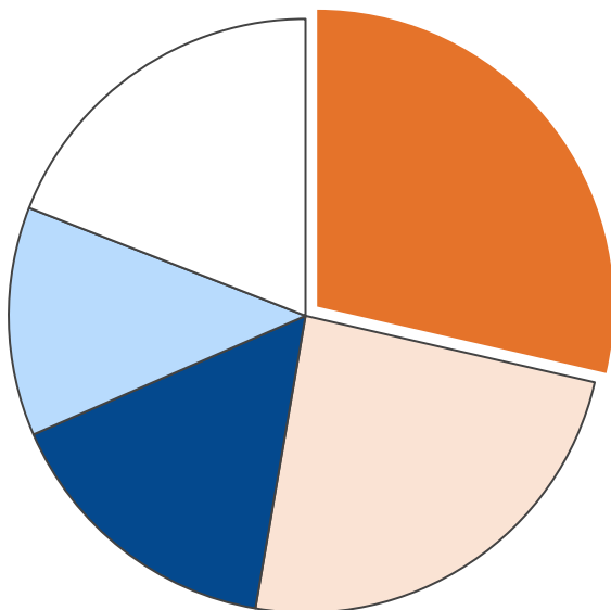
産業部門・エネルギー消費量合計 5,413 TJ
