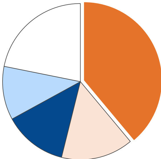
産業部門・エネルギー消費量合計 2,631 TJ
