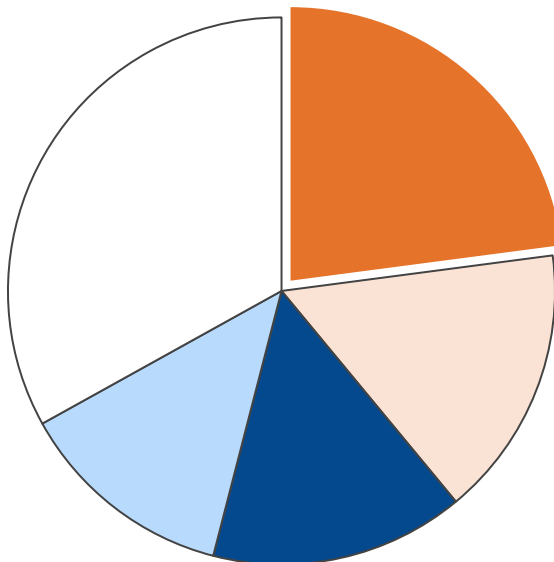
業務部門・エネルギー消費量合計 2,358 TJ
