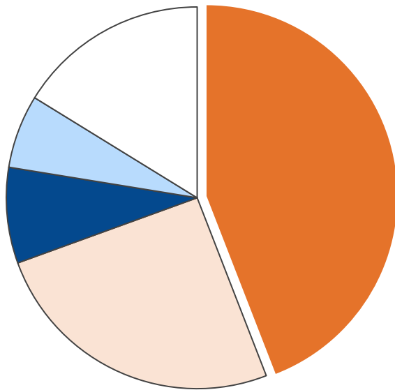
産業部門・二酸化炭素排出量合計 165,712 t-CO 2
