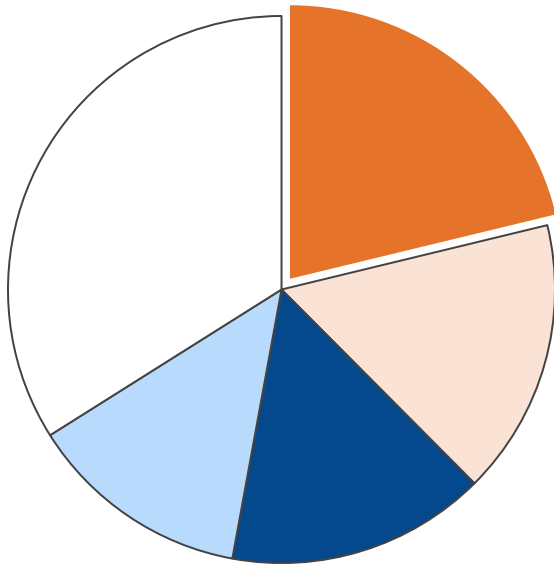
業務部門・二酸化炭素排出量合計 97,090 t-CO 2
