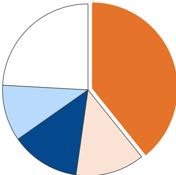
産業部門・エネルギー消費量合計 107 TJ
