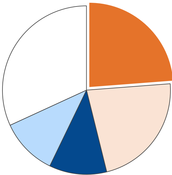
業務部門・二酸化炭素排出量合計 9,403 t-CO 2
