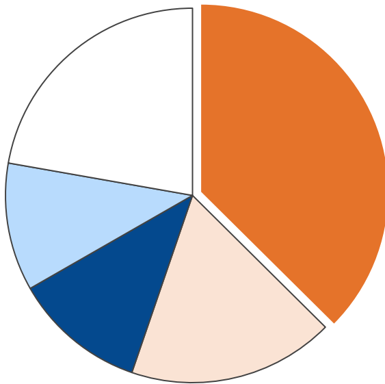
産業部門・二酸化炭素排出量合計 7,694 t-CO 2
