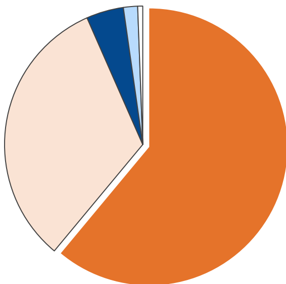
産業部門・二酸化炭素排出量合計 115,630 t-CO 2
