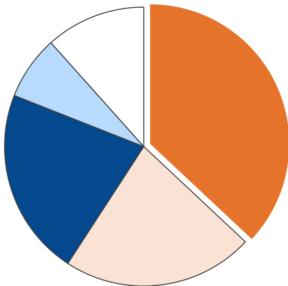
産業部門・二酸化炭素排出量合計 151,225 t-CO 2
