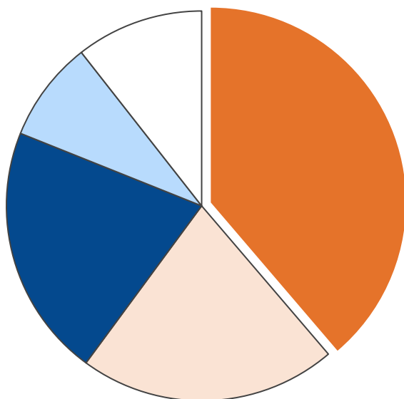
産業部門・エネルギー消費量合計 3,402 TJ
