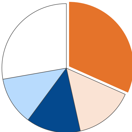
業務部門・エネルギー消費量合計 680 TJ
