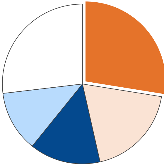
業務部門・二酸化炭素排出量合計 29,344 t-CO 2
