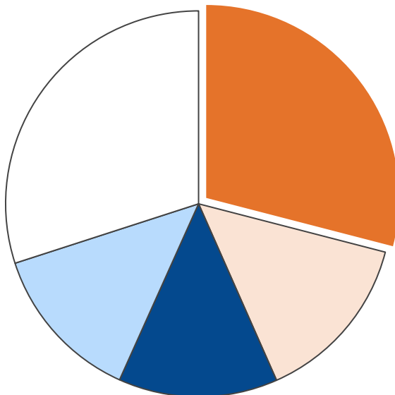
業務部門・エネルギー消費量合計 130 TJ
