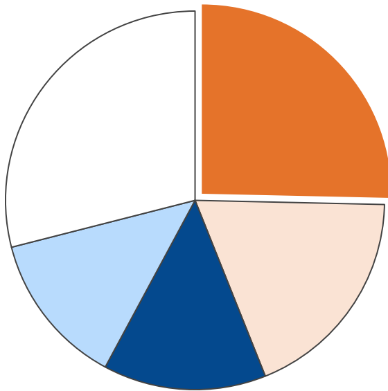
業務部門・二酸化炭素排出量合計 5,598 t-CO 2
