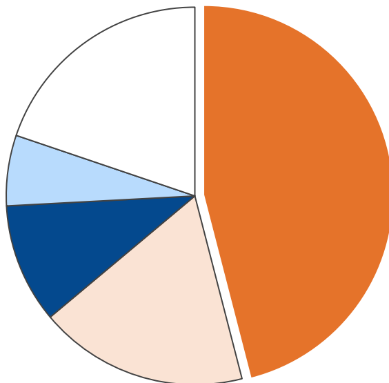
産業部門・エネルギー消費量合計 453 TJ
