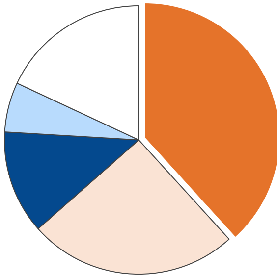
産業部門・二酸化炭素排出量合計 20,705 t-CO 2
