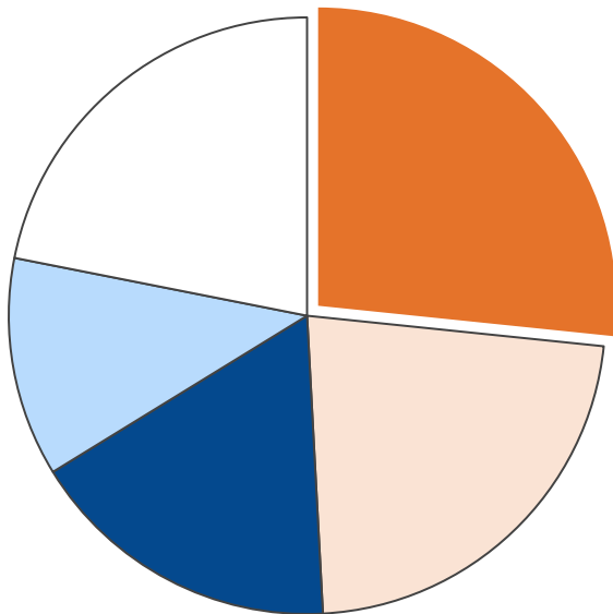
業務部門・二酸化炭素排出量合計 5,751 t-CO 2
