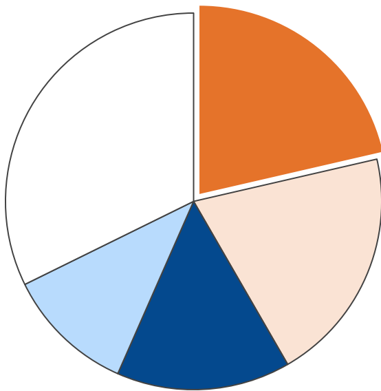
業務部門・二酸化炭素排出量合計 1,248 t-CO 2
