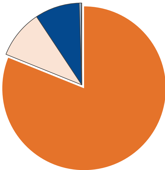
産業部門・二酸化炭素排出量合計 3,640 t-CO 2
