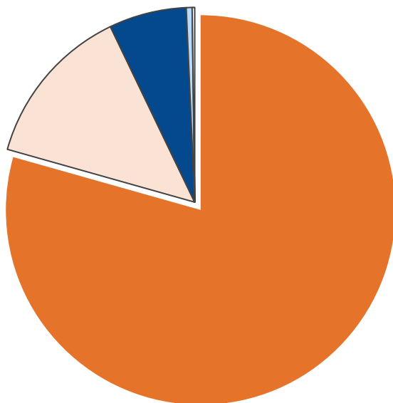
産業部門・エネルギー消費量合計 57 TJ
