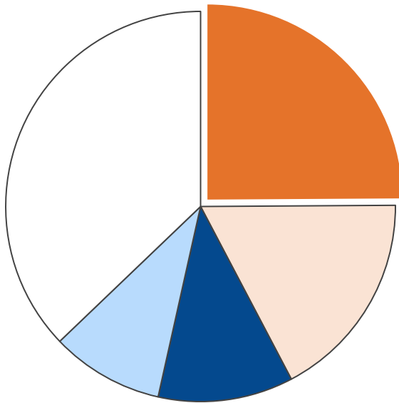
業務部門・二酸化炭素排出量合計 4,938 t-CO 2
