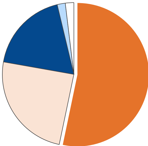
産業部門・二酸化炭素排出量合計 16,174 t-CO 2
