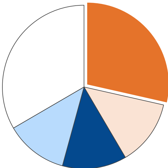
業務部門・エネルギー消費量合計 192 TJ
