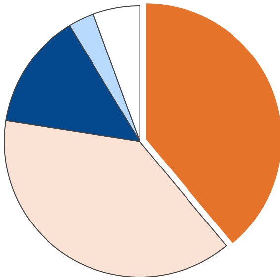
産業部門・二酸化炭素排出量合計 31,095 t-CO 2
