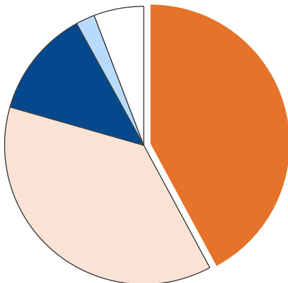
産業部門・エネルギー消費量合計 457 TJ
