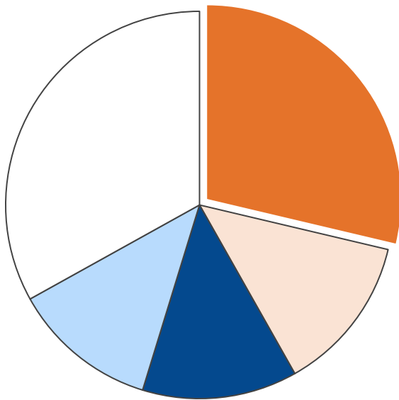
業務部門・二酸化炭素排出量合計 12,211 t-CO 2
