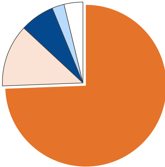
産業部門・二酸化炭素排出量合計 26,019 t-CO 2
