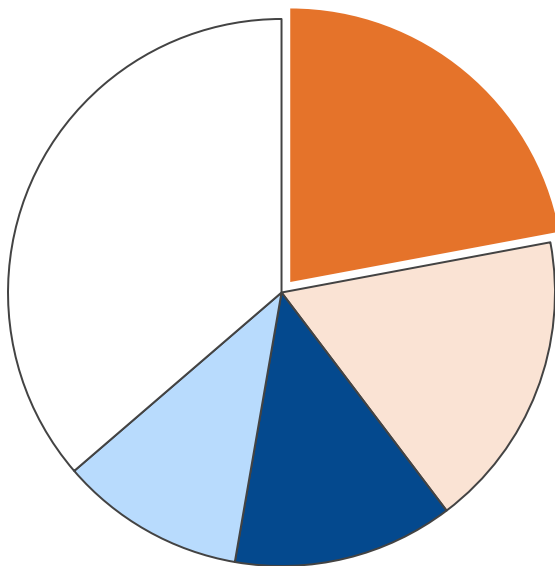
業務部門・二酸化炭素排出量合計 5,275 t-CO 2
