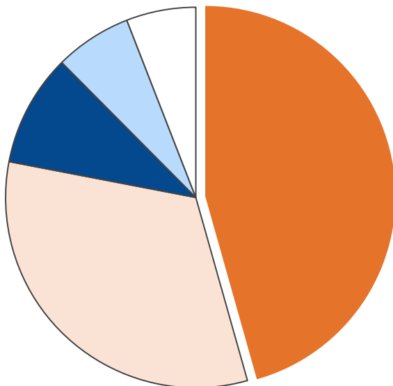
産業部門・エネルギー消費量合計 577 TJ
