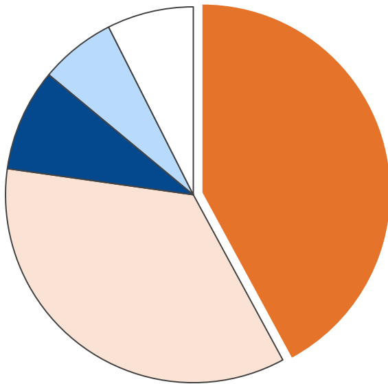
産業部門・二酸化炭素排出量合計 36,900 t-CO 2
