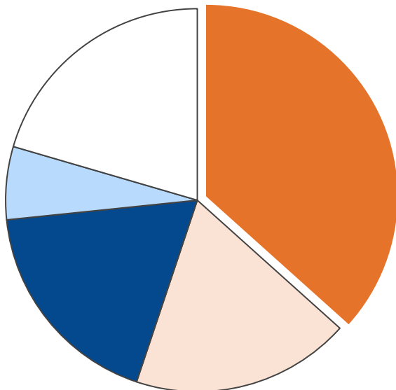
業務部門・エネルギー消費量合計 199 TJ
