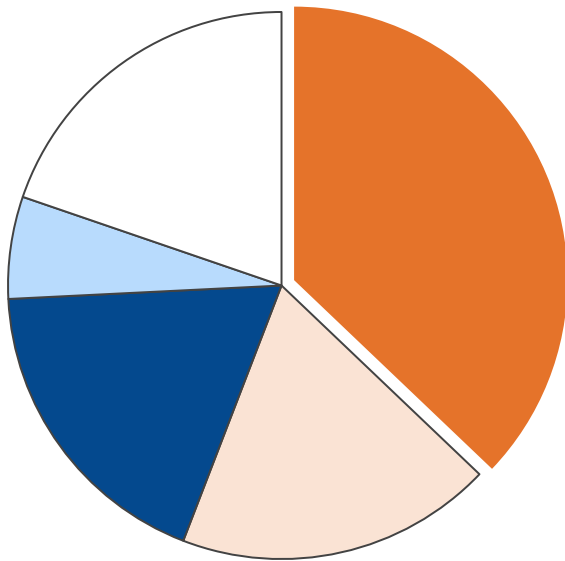
業務部門・二酸化炭素排出量合計 11,748 t-CO 2
