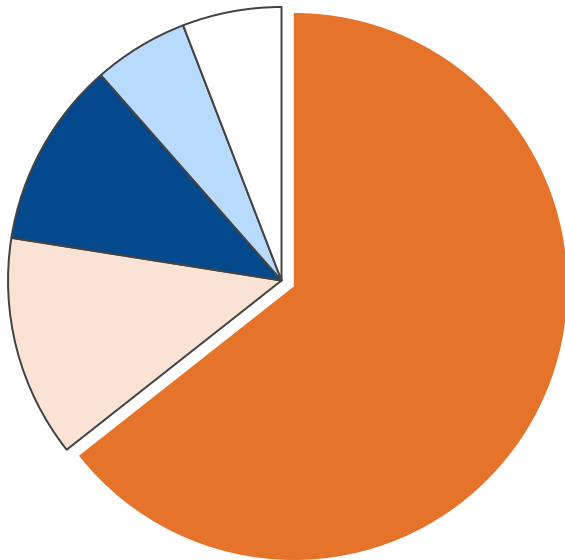
産業部門・二酸化炭素排出量合計 2,458 t-CO 2
