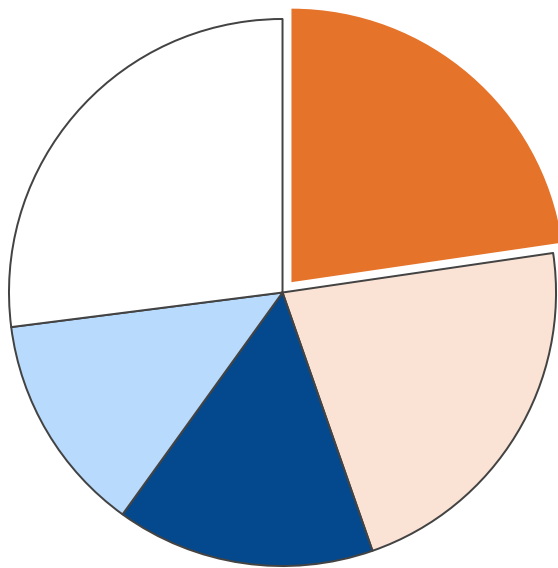
業務部門・二酸化炭素排出量合計 2,929 t-CO 2
