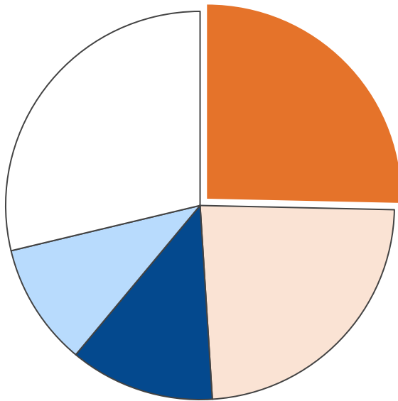
業務部門・二酸化炭素排出量合計 2,103 t-CO 2
