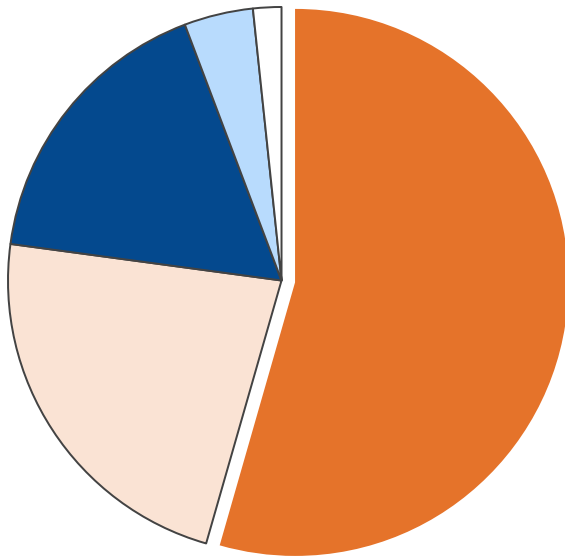
産業部門・二酸化炭素排出量合計 5,757 t-CO 2
