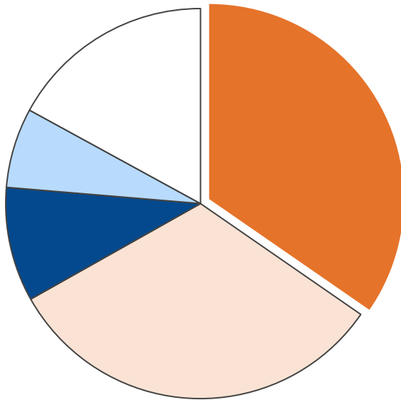
産業部門・二酸化炭素排出量合計 208,859 t-CO 2
