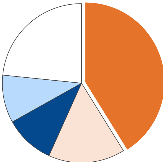
産業部門・エネルギー消費量合計 2,568 TJ
