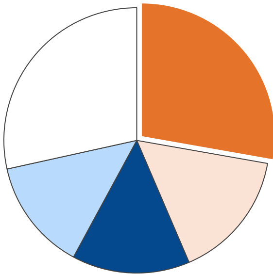
業務部門・二酸化炭素排出量合計 87,436 t-CO 2
