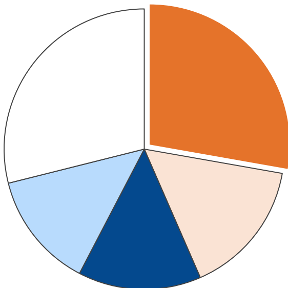
業務部門・エネルギー消費量合計 1,580 TJ
