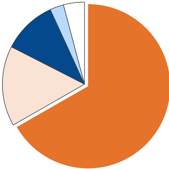
産業部門・二酸化炭素排出量合計 201,950 t-CO 2
