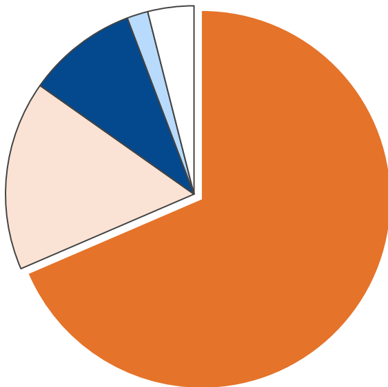
産業部門・エネルギー消費量合計 3,534 TJ
