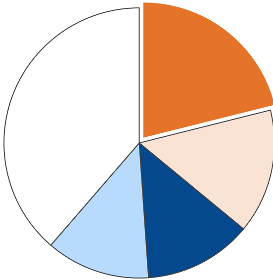
業務部門・二酸化炭素排出量合計 138,388 t-CO 2
