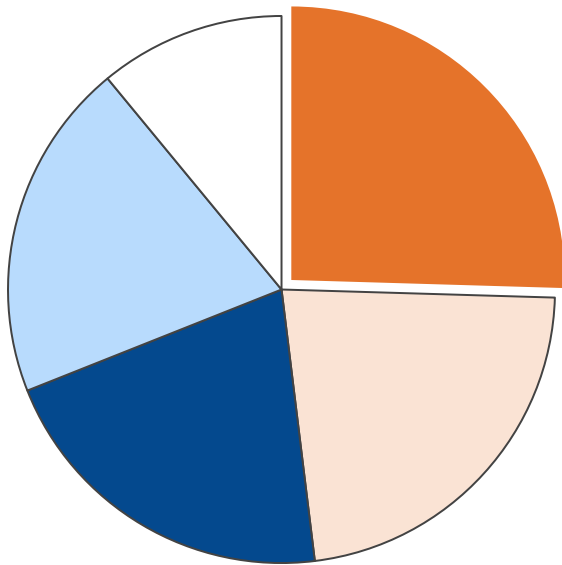
産業部門・二酸化炭素排出量合計 7,553 t-CO 2
