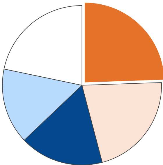
業務部門・二酸化炭素排出量合計 4,861 t-CO 2
