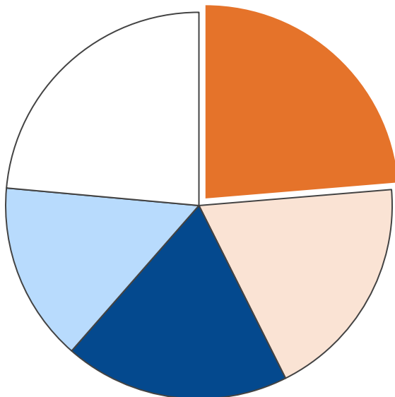
業務部門・エネルギー消費量合計 716 TJ
