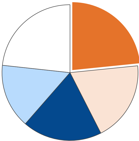
業務部門・二酸化炭素排出量合計 39,941 t-CO 2
