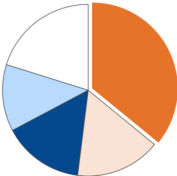
産業部門・二酸化炭素排出量合計 33,847 t-CO2
