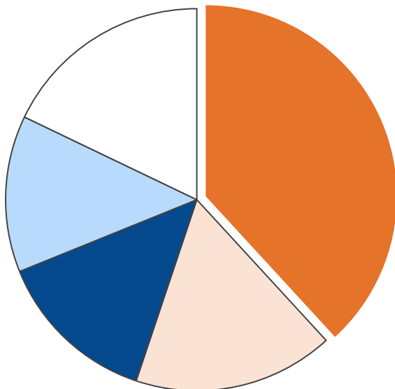
産業部門・エネルギー消費量合計 575 TJ
