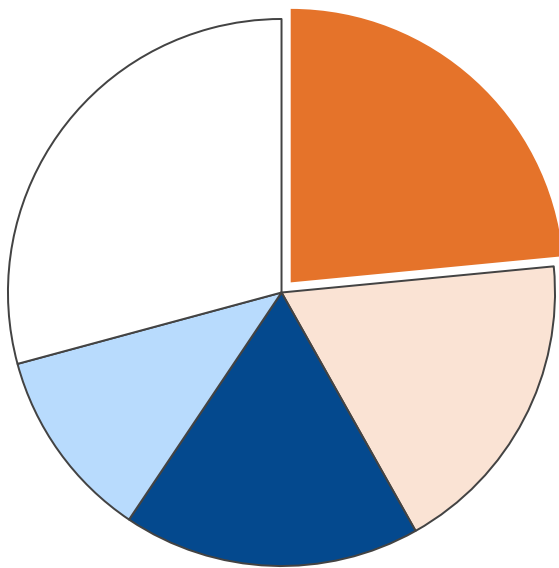
業務部門・二酸化炭素排出量合計 9,294 t-CO 2
