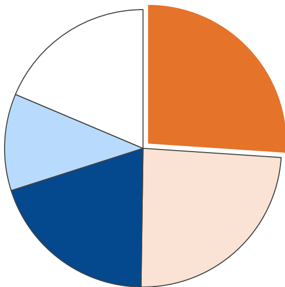
産業部門・二酸化炭素排出量合計 40,028 t-CO 2
