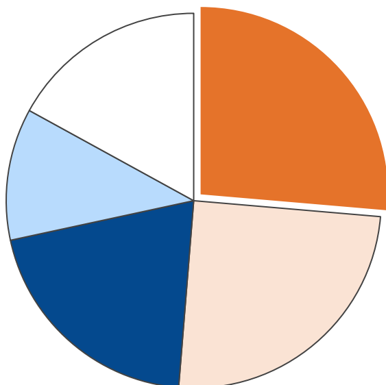
産業部門・エネルギー消費量合計 716 TJ
