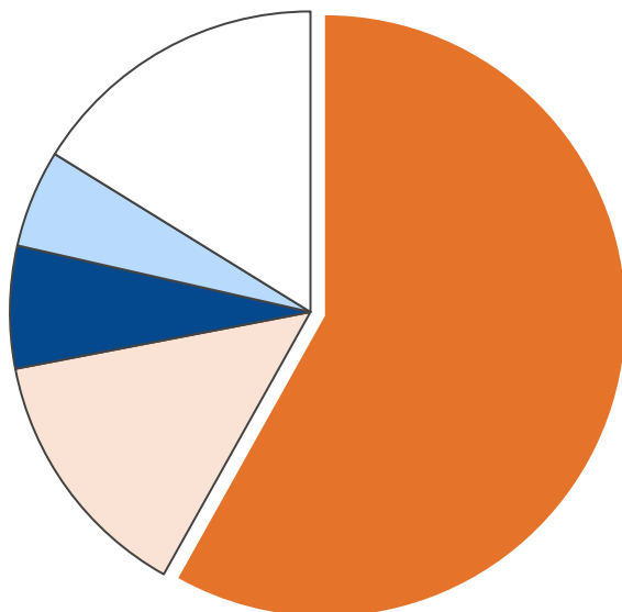
産業部門・エネルギー消費量合計 7,022 TJ
