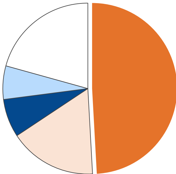
産業部門・二酸化炭素排出量合計 322,211 t-CO 2
