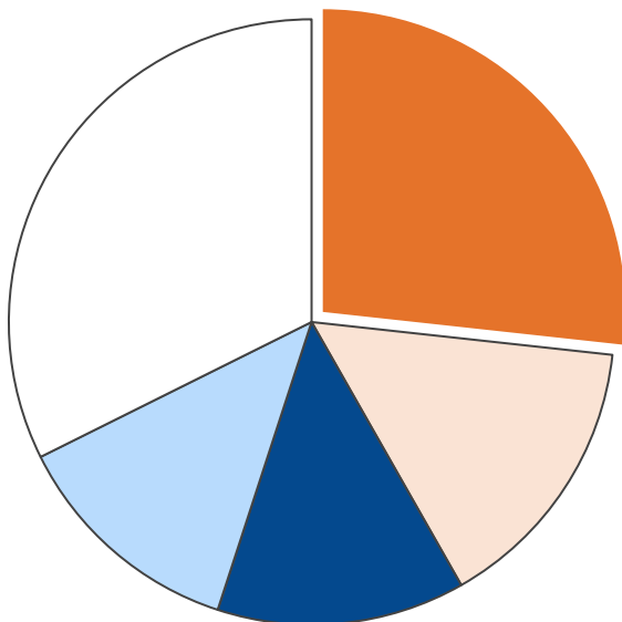
業務部門・エネルギー消費量合計 1,887 TJ
