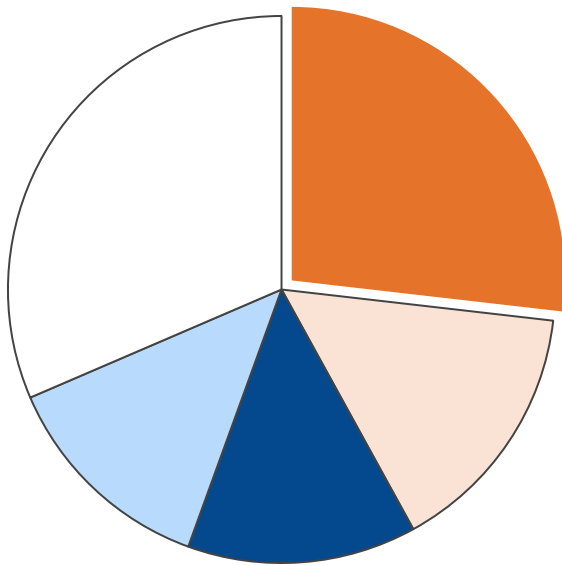
業務部門・二酸化炭素排出量合計 103,398 t-CO 2
