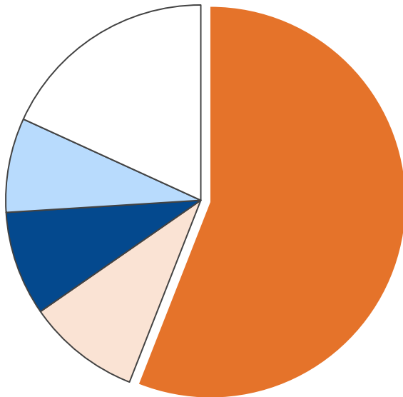
産業部門・二酸化炭素排出量合計 77,604 t-CO2
