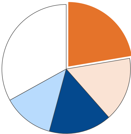
業務部門・二酸化炭素排出量合計 8,061 t-CO 2
