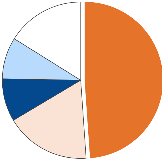
産業部門・二酸化炭素排出量合計 10,036 t-CO 2
