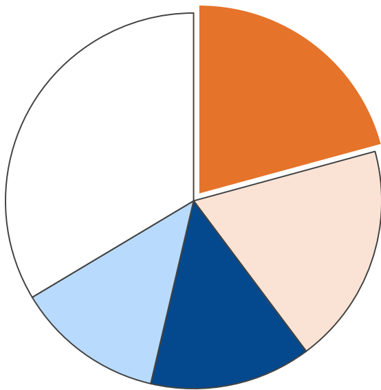
業務部門・二酸化炭素排出量合計 19,149 t-CO2
