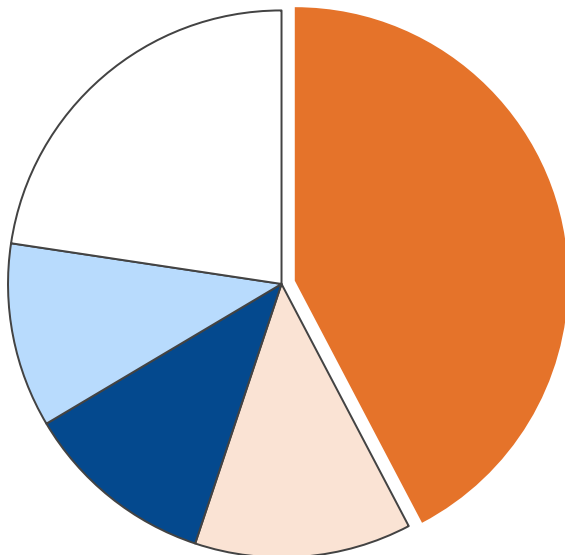
産業部門・エネルギー消費量合計 178 TJ
