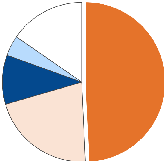
産業部門・エネルギー消費量合計 4,085 TJ
