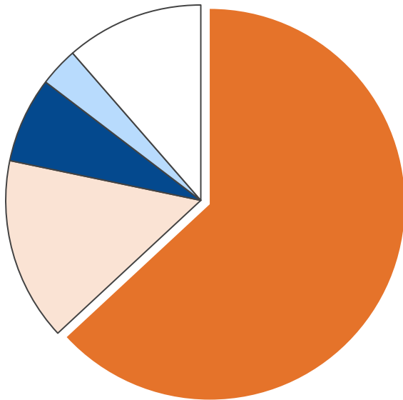
産業部門・二酸化炭素排出量合計 337,933 t-CO 2
