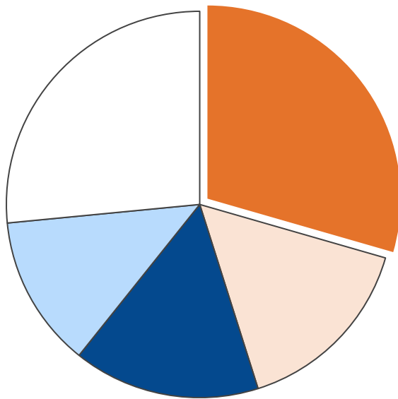
業務部門・二酸化炭素排出量合計 135,346 t-CO 2
