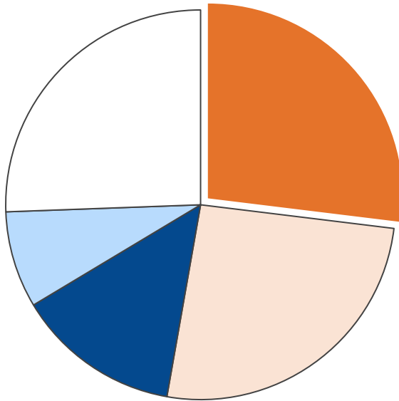
業務部門・二酸化炭素排出量合計 223,548 t-CO 2
