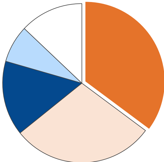
産業部門・エネルギー消費量合計 10,390 TJ
