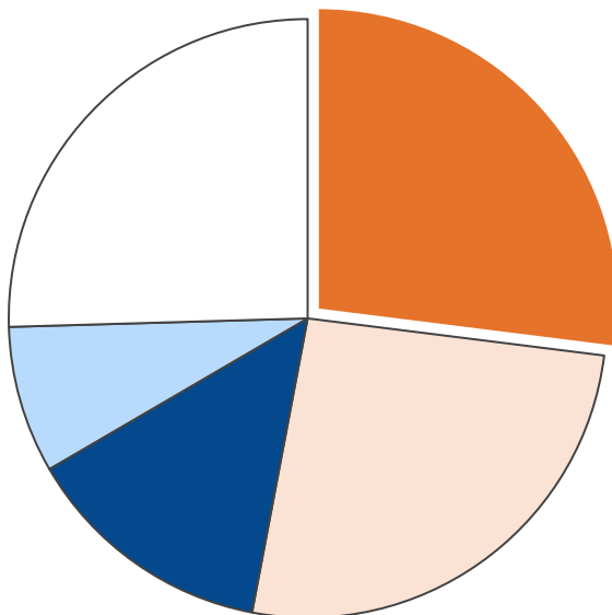
業務部門・エネルギー消費量合計 3,824 TJ
