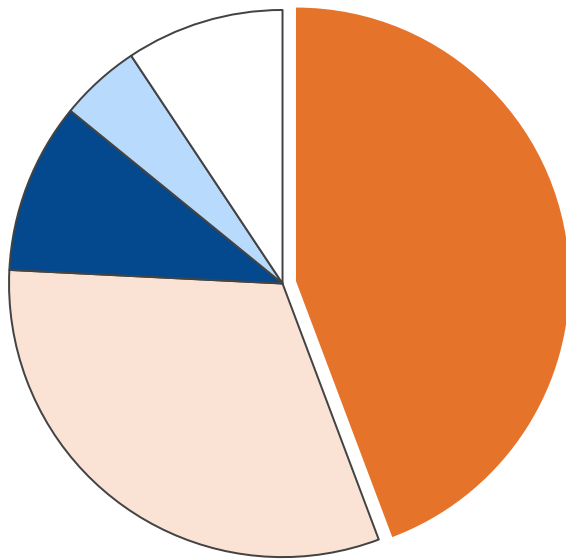
産業部門・二酸化炭素排出量合計 921,054 t-CO 2
