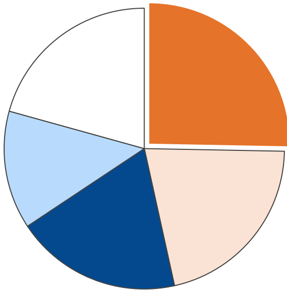
業務部門・二酸化炭素排出量合計 6,715 t-CO 2
