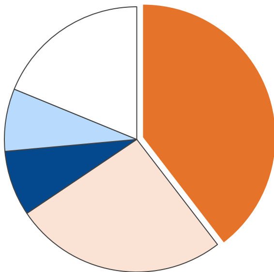
産業部門・二酸化炭素排出量合計 17,318 t-CO 2
