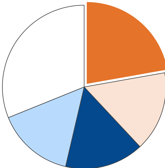
業務部門・エネルギー消費量合計 1,656 TJ
