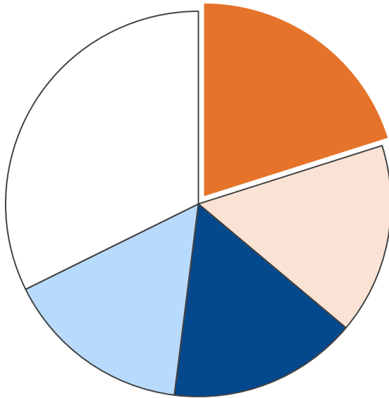
業務部門・二酸化炭素排出量合計 68,806 t-CO 2
