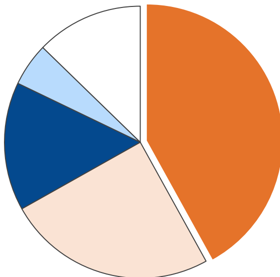
産業部門・エネルギー消費量合計 703 TJ
