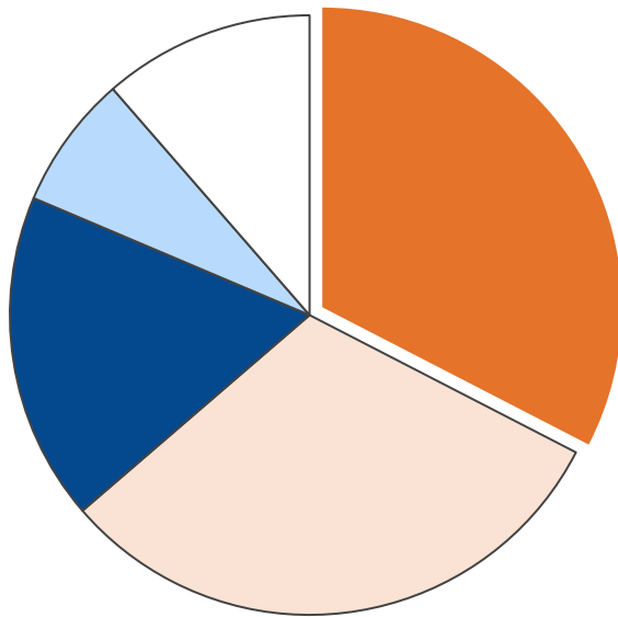
産業部門・二酸化炭素排出量合計 39,977 t-CO 2
