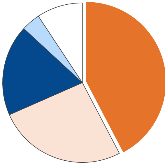
産業部門・二酸化炭素排出量合計 19,933 t-CO 2
