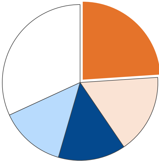
業務部門・二酸化炭素排出量合計 52,784 t-CO2
