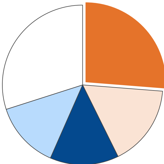
業務部門・エネルギー消費量合計 1,280 TJ
