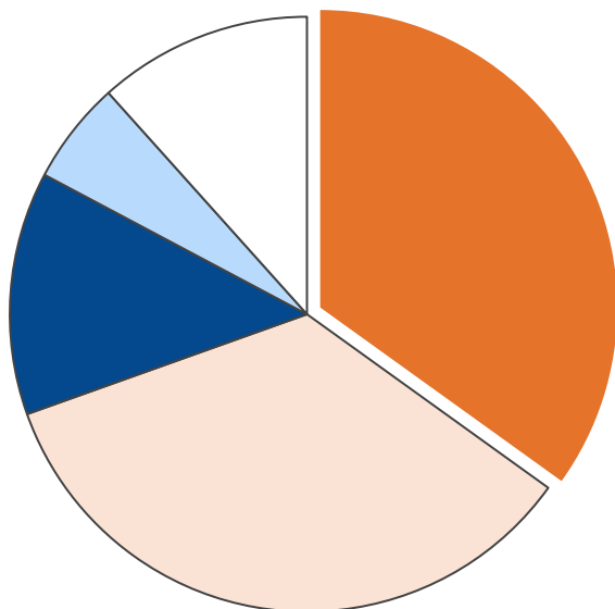
産業部門・エネルギー消費量合計 340 TJ
