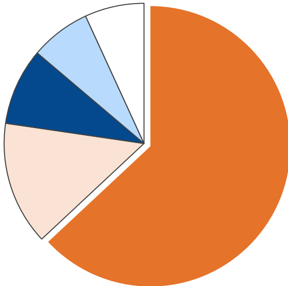
産業部門・エネルギー消費量合計 16 TJ
