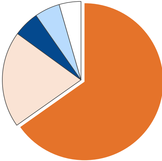
産業部門・二酸化炭素排出量合計 1,019 t-CO 2
